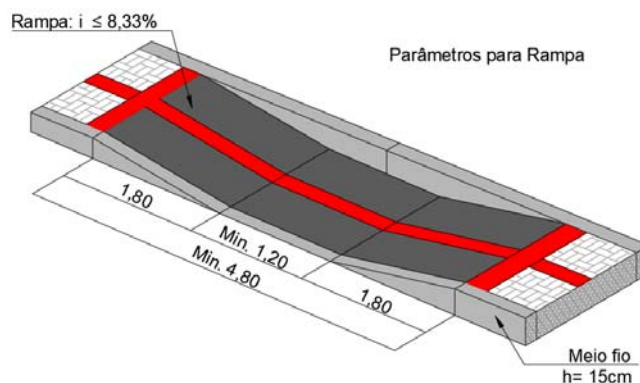
Figura 24 – Detalhe da rampa de acessibilidade
