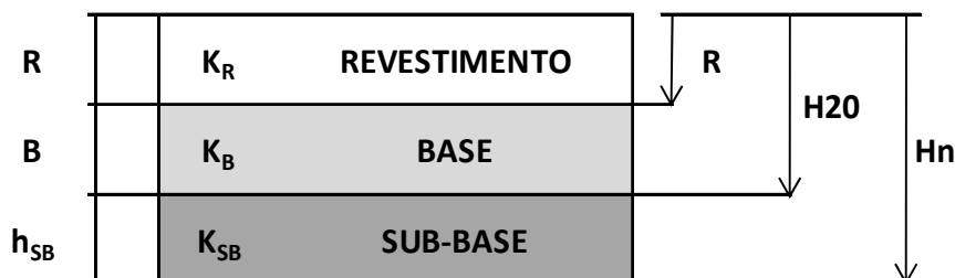
Figura 12 – Representação das camadas estruturais do pavimento
