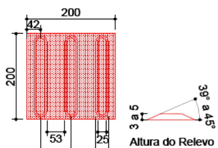
SINALIZAÇÃO TÁTIL DE DIRECIONAL
