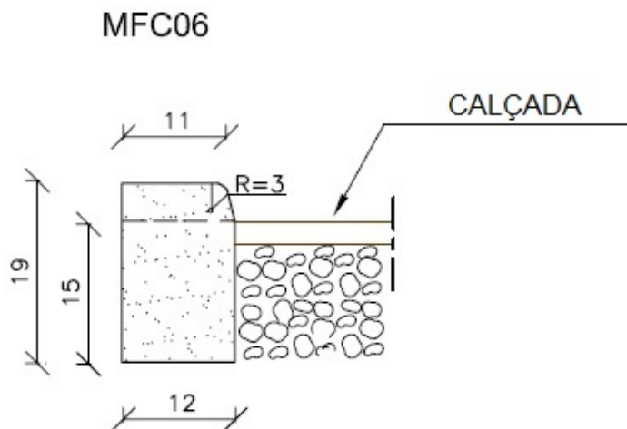
Figura 21 – Meio-fio tipo 6 de travamento/reto
