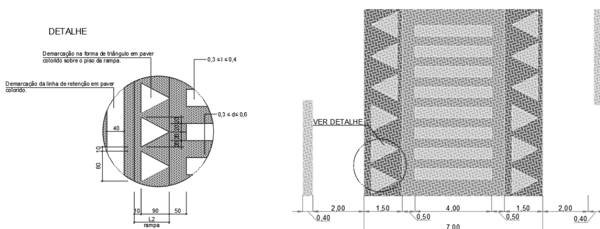
Figura 22 – Detalhe da faixa elevada
