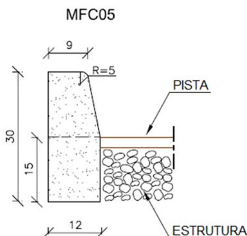
Figura 20 – Meio-fio tipo 5
