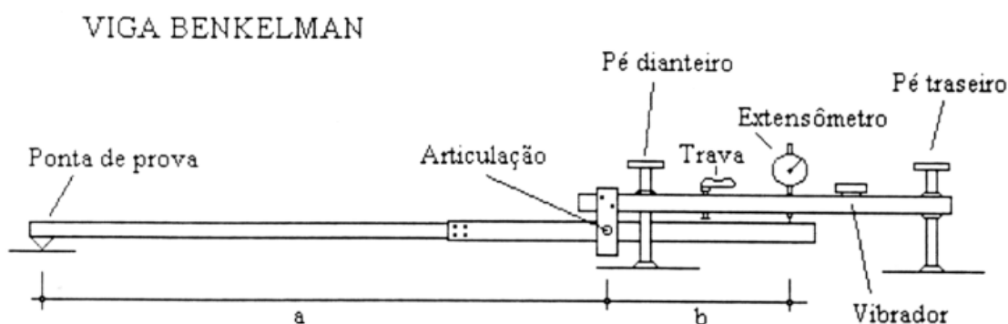
Figura 8 – Esquema da viga Benkelman
