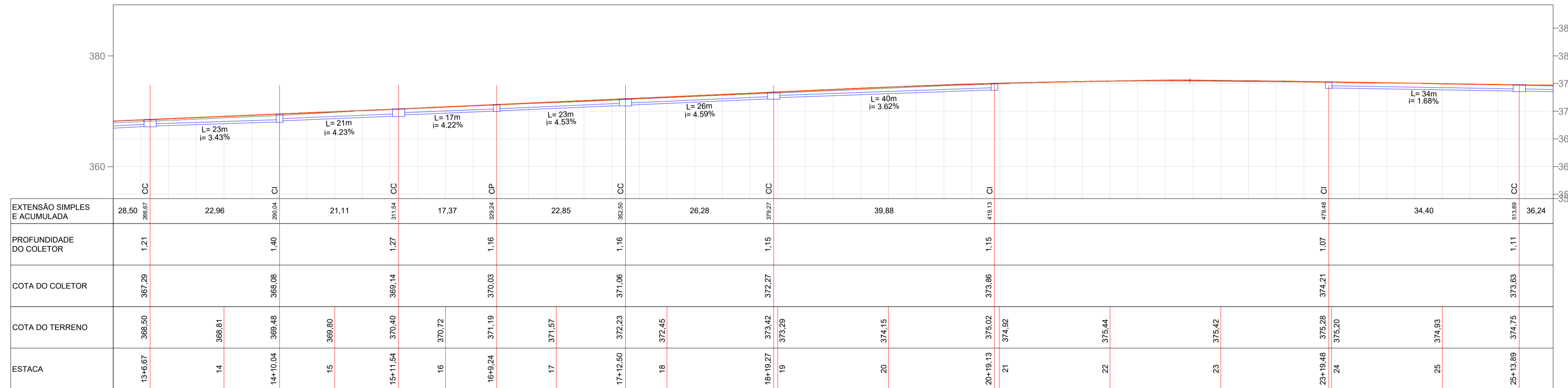
Perfil Drenagem - Lado Direito Est: 13 + 0,00 à 26 + 0,00 Esc: 1/500
