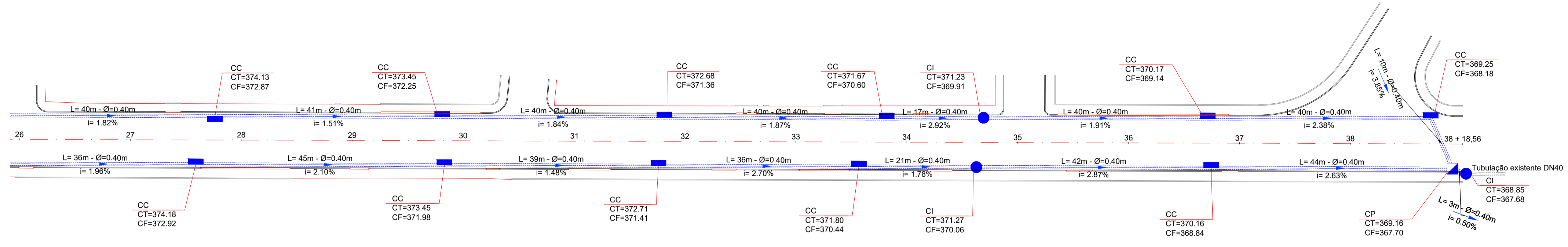
Planta Baixa Est: 26 + 0,00 à 38 + 18,56 Esc: 1/500
