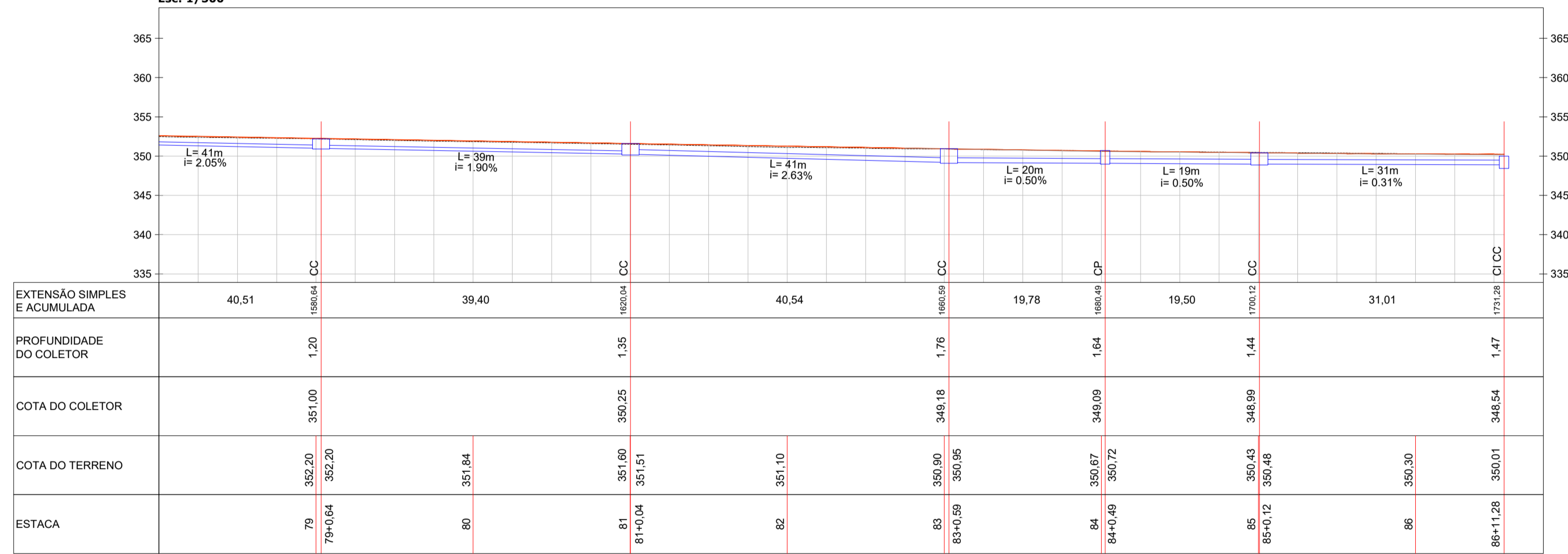
Perfil Drenagem - Avenida Nereu Ramos (Lado Direito) Est: 78 + 0,00 à 86 + 11,33 Esc: 1/500
