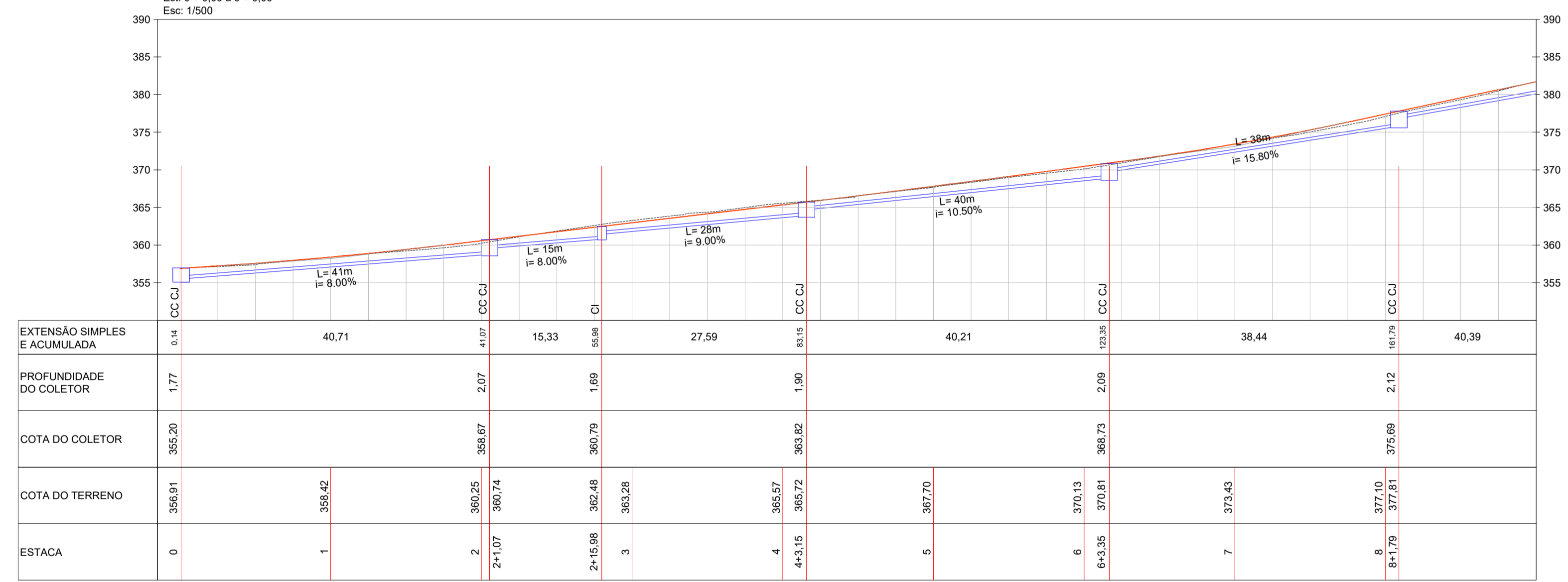
Perfil - Drenagem (Lado Direito) Est: 0 + 0,00 à 9 + 0,00 Esc: 1/500
