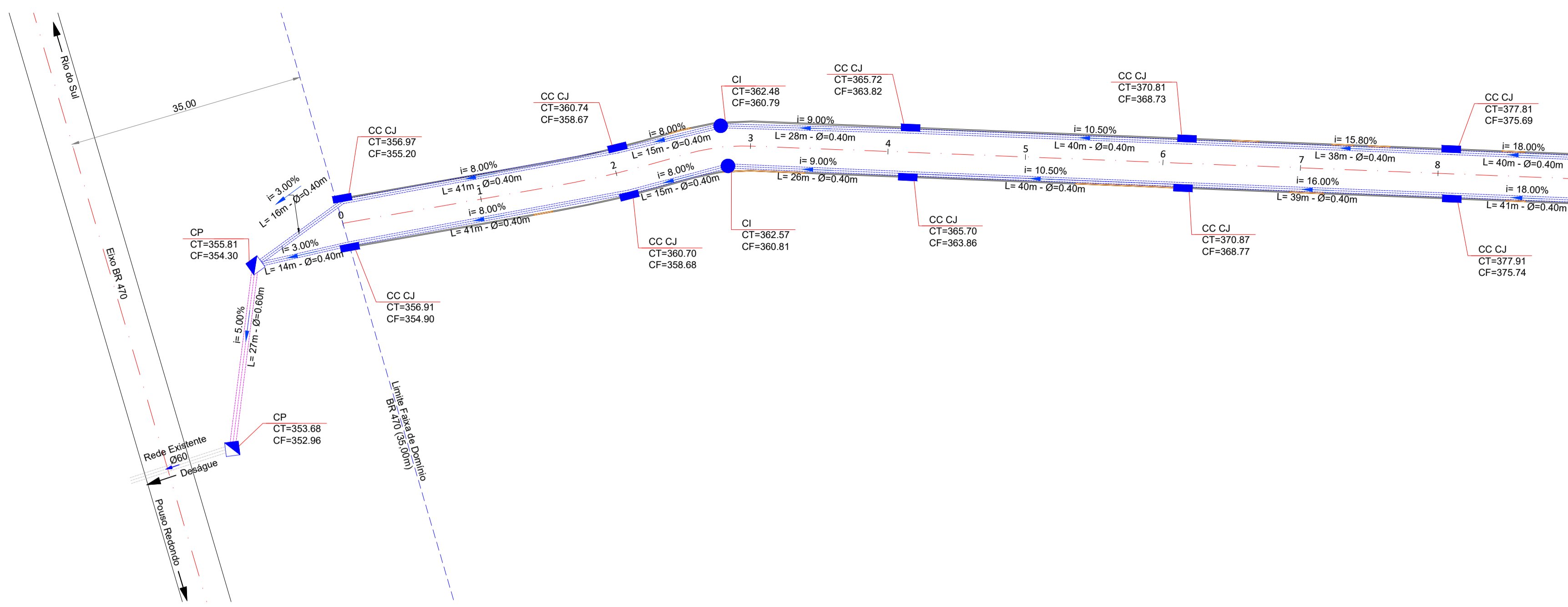
Planta Baixa Est: 0 + 0,00 à 9 + 0,00 Esc: 1/500
