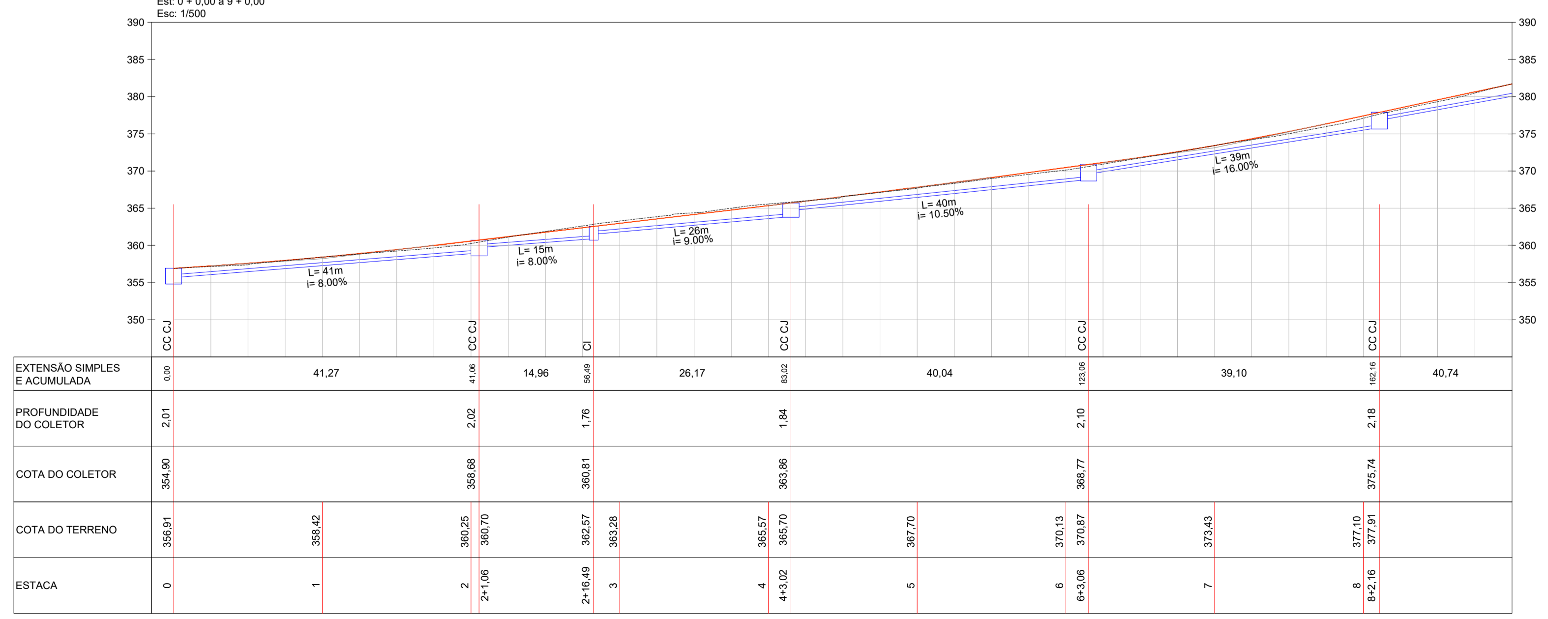
Perfil - Drenagem (Lado Direito) Est: 0 + 0,00 à 9 + 0,00 Esc: 1/500
