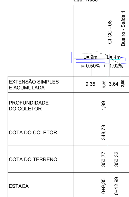
Perfil Drenagem - Rua Ernesto Prada Saída 1 Esc: 1/500
