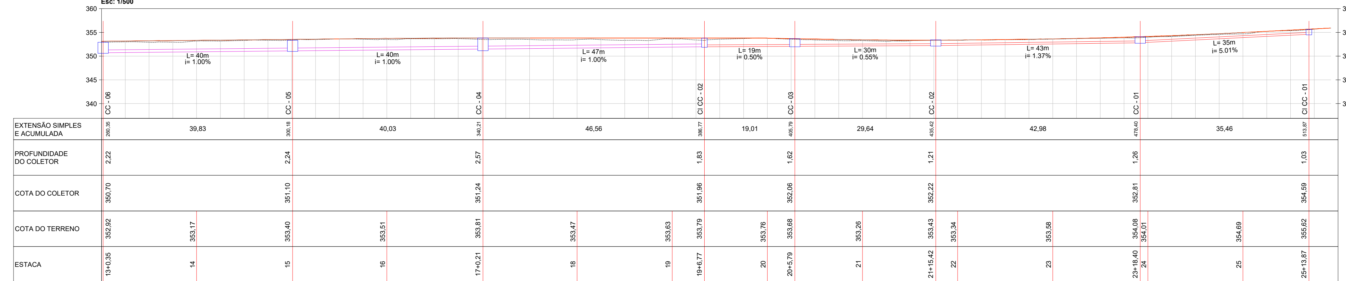
Perfil Drenagem - Rua Ernesto Prada (Lado Esquerdo) Est: 13 + 0,00 à 25 + 18,60 Esc: 1/500
